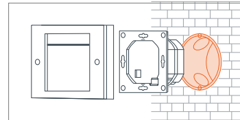
Installation af styreenhed og læserenhed i en indbygget boks
